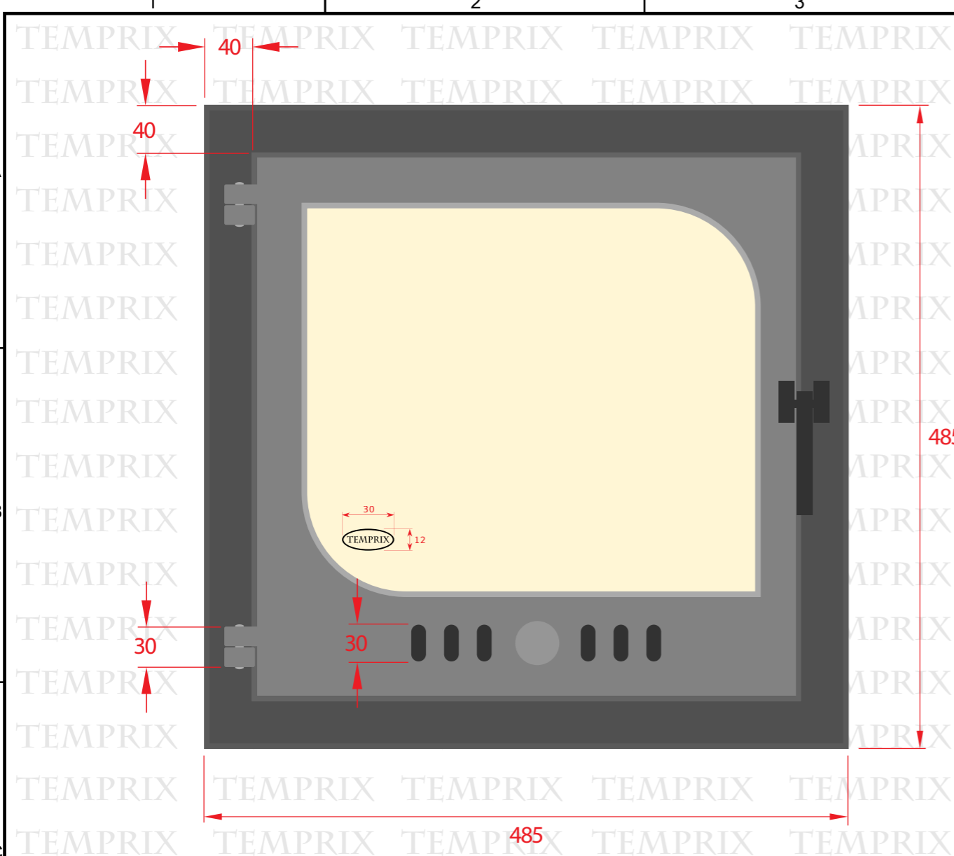
Frontansicht
