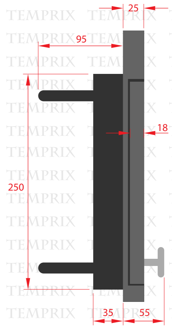
Seitenansicht
